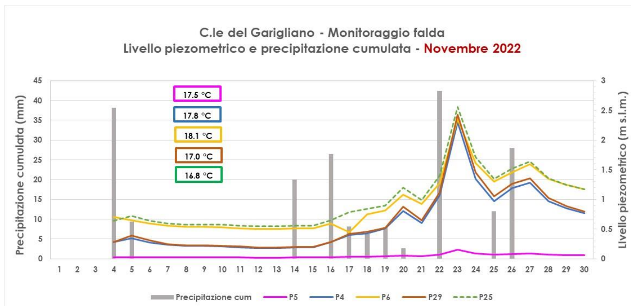
Figura 5.9 Andamento del livello piezometrico nei 5 piezometri e della precipitazione cumulata - Novembre 2022
