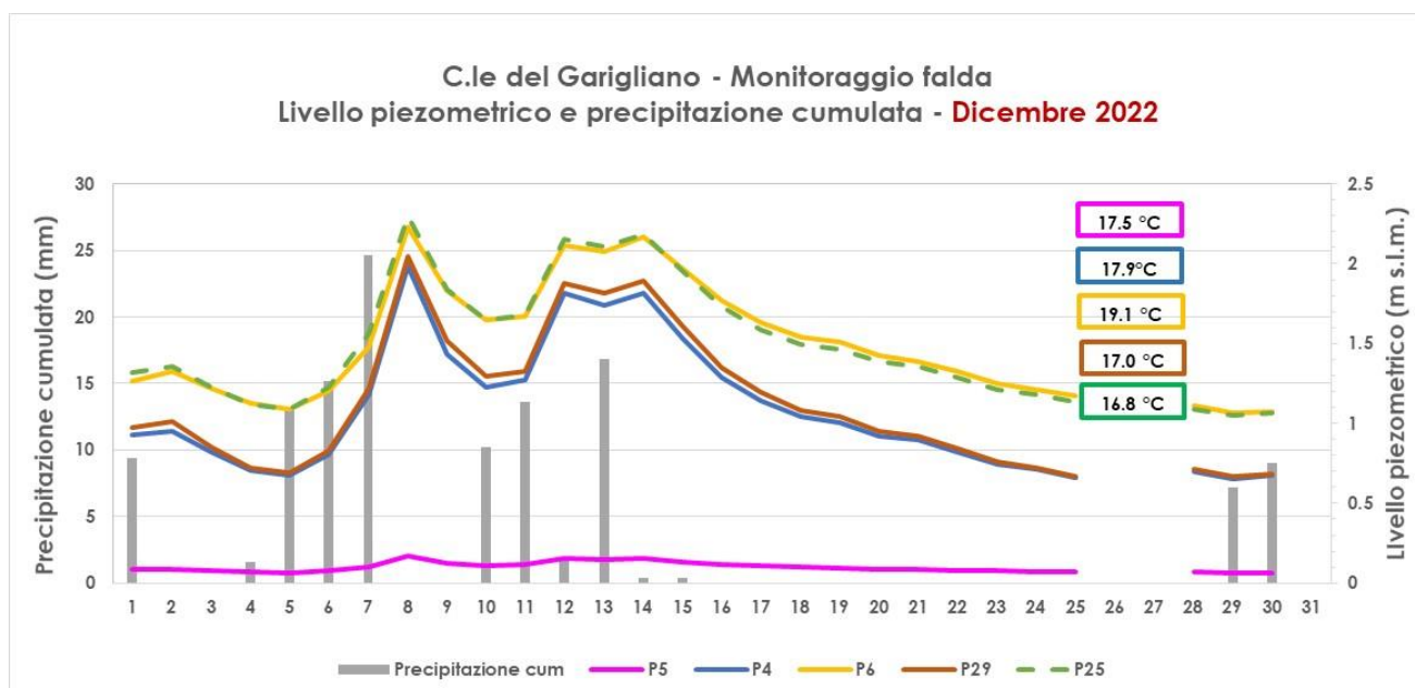
Figura 5.10 Andamento del livello piezometrico nei 5 piezometri e della precipitazione cumulata - Dicembre 2022
