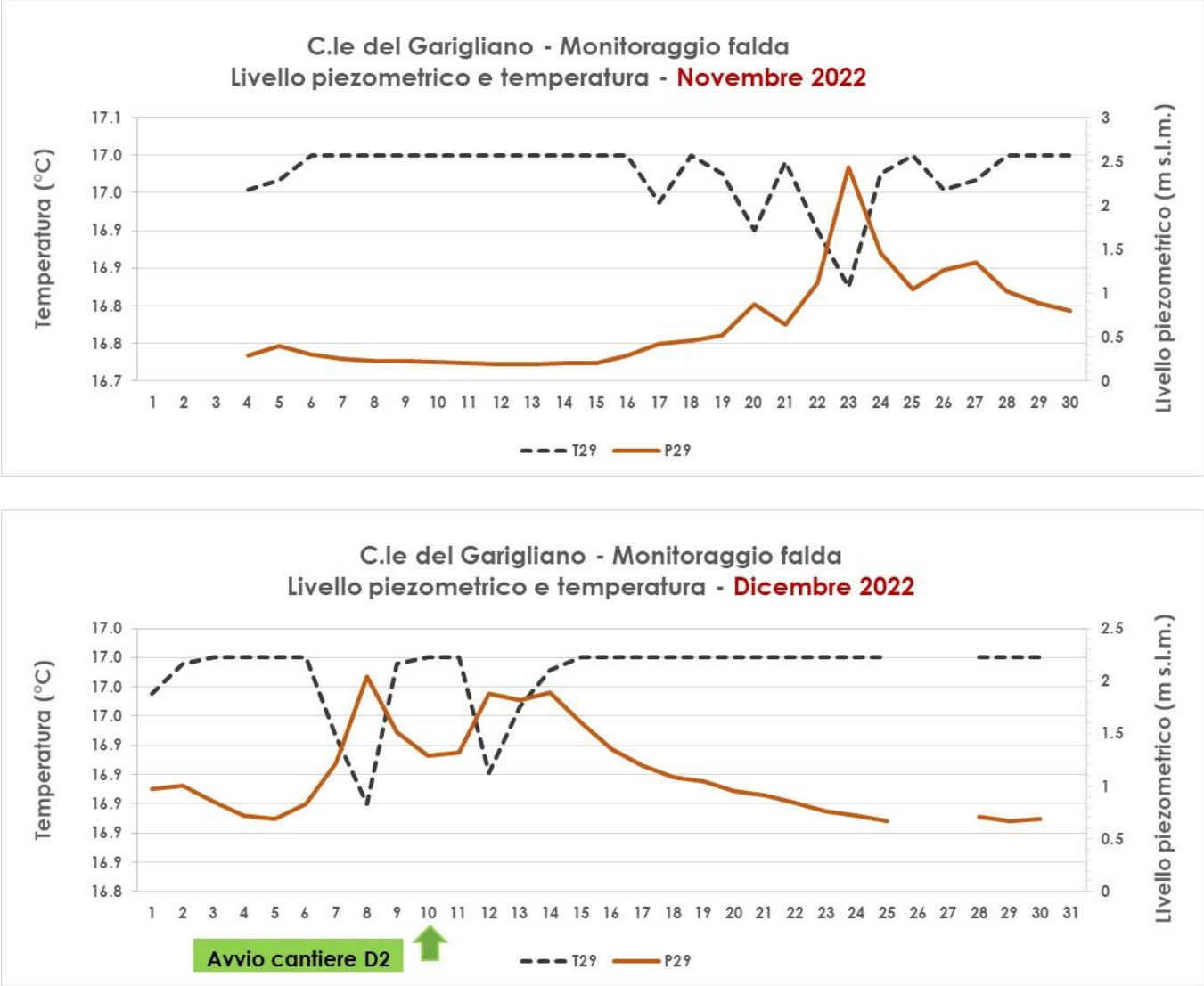
Figura 5.14 Andamento del livello piezometrico e della temperatura nei mesi di novembre e dicembre 2022 - Piezometro P29
