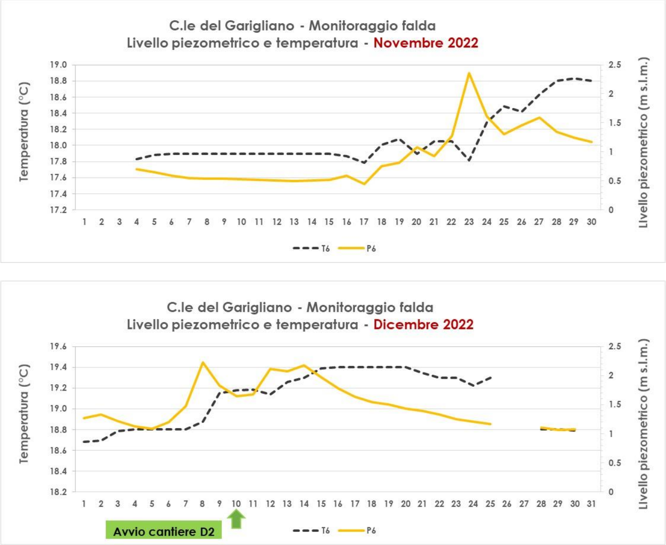
Figura 5.13 Andamento del livello piezometrico e della temperatura nei mesi di novembre e dicembre 2022 - Piezometro P6
