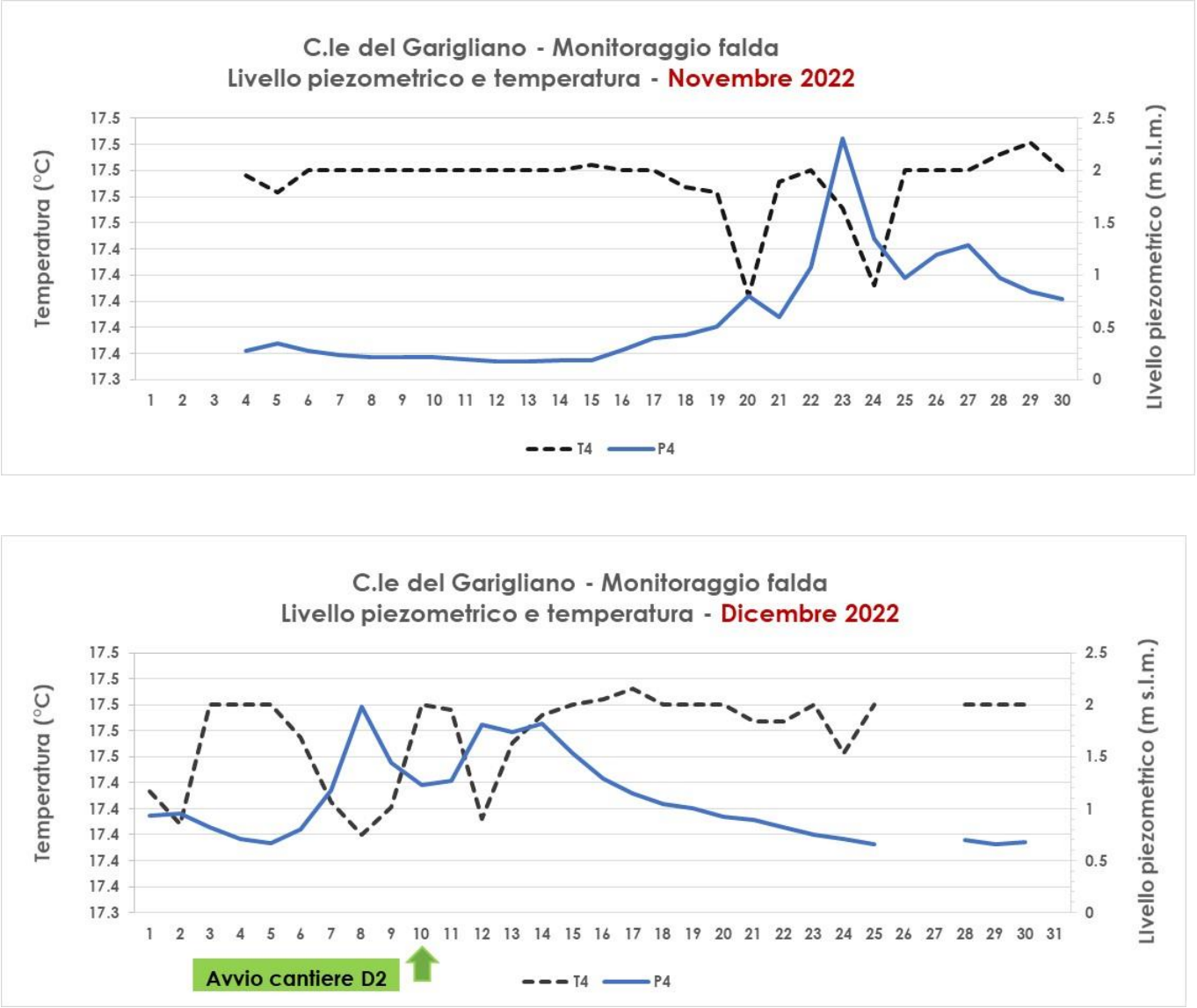
Figura 5.11 Andamento del livello piezometrico e della temperatura nei mesi di novembre e dicembre 2022 - Piezometro P4
