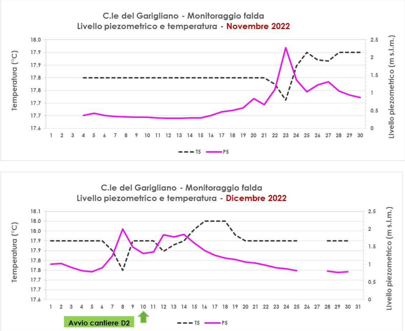
Figura 5.12 Andamento del livello piezometrico e della temperatura nei mesi di novembre e dicembre 2022 - Piezometro P5
