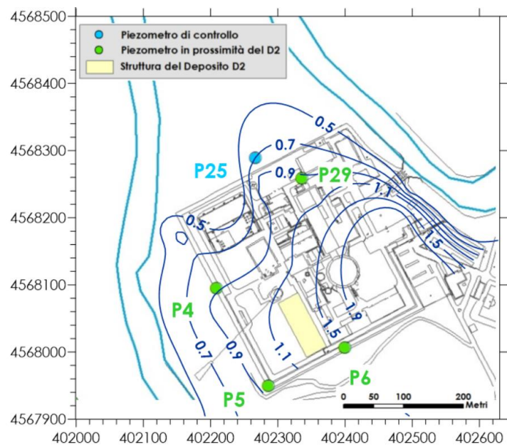
Figura 5.8 Ubicazione dei punti di misura per il monitoraggio in continuo
