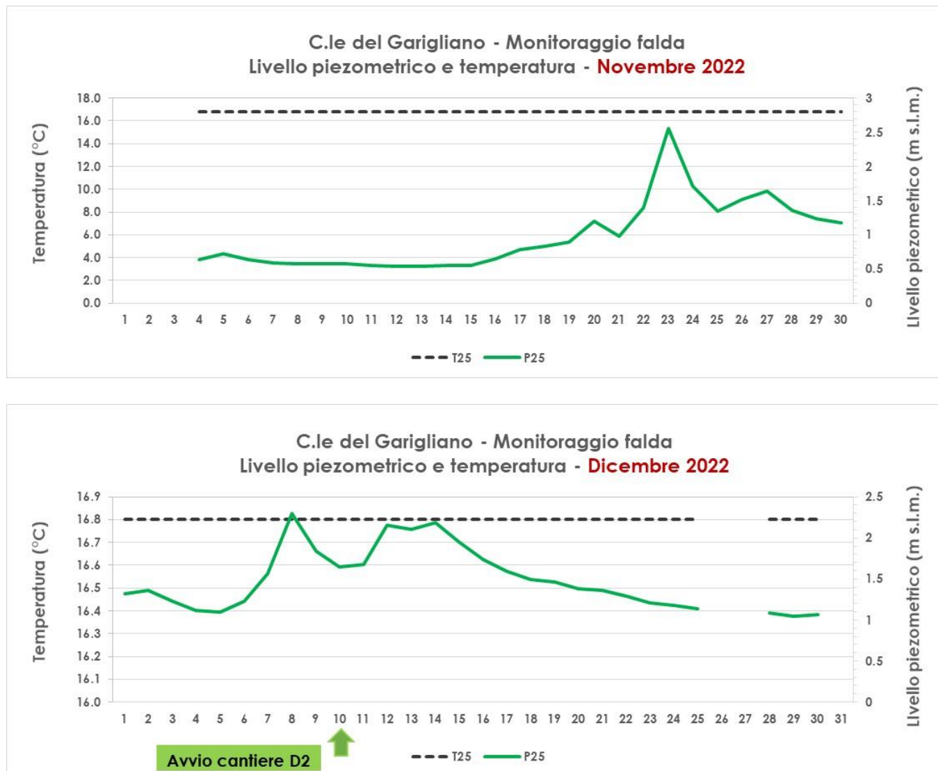
Figura 5.15 Andamento del livello piezometrico e della temperatura nei mesi di novembre e dicembre 2022 - Piezometro P25
